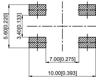
Welding diagram 焊接图
