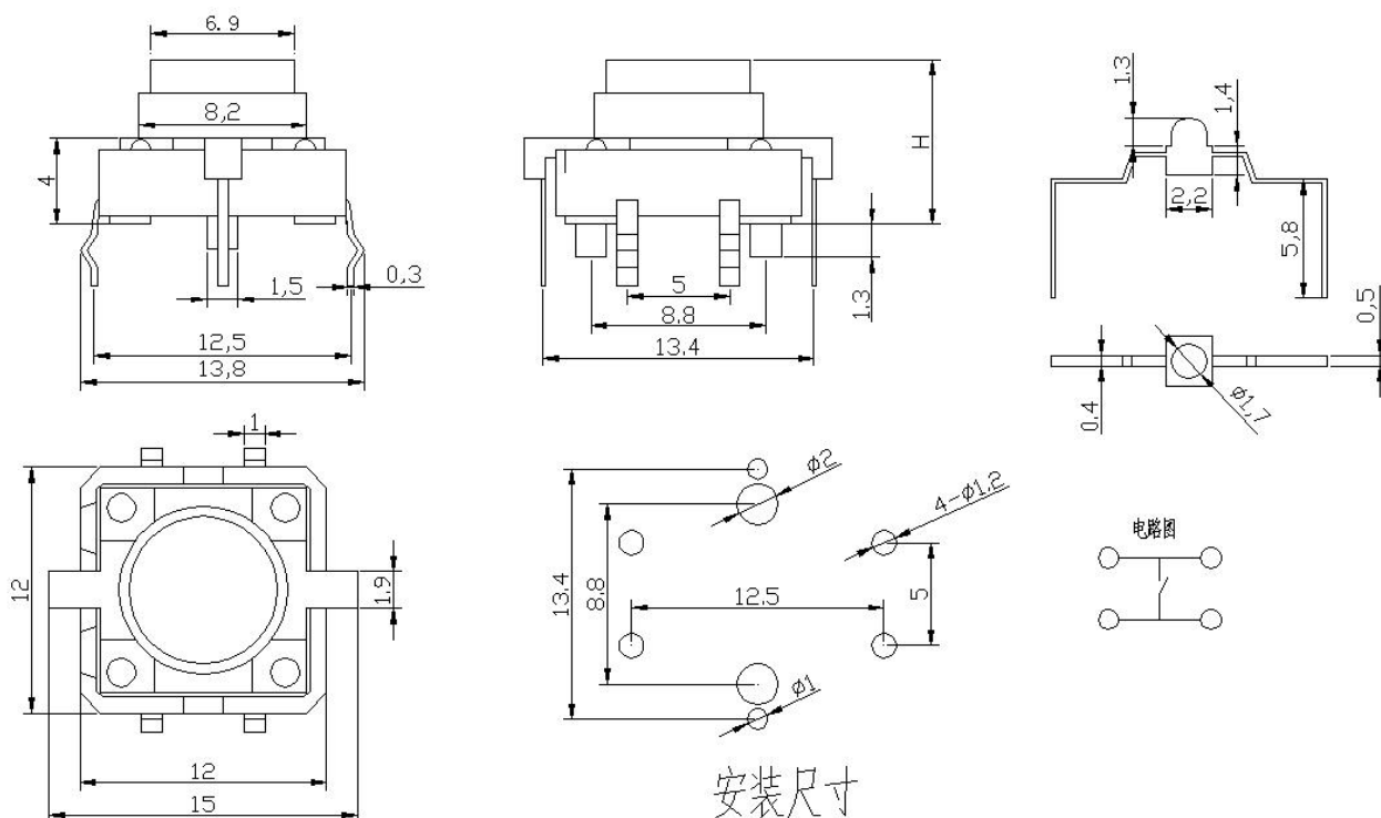
尺寸外型图
