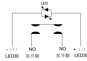
Schematic Diagram 电气原理图
