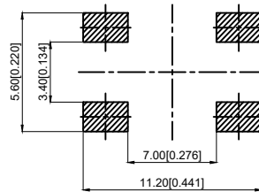
PCB LAND DIMENSION PCB电路板焊盘尺寸
