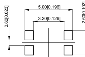
PCB.安装尺寸图
