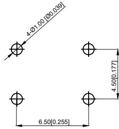
PCB.焊接图
