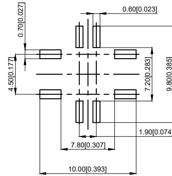
PCB. Installation diagram PCB. 安装示意图
