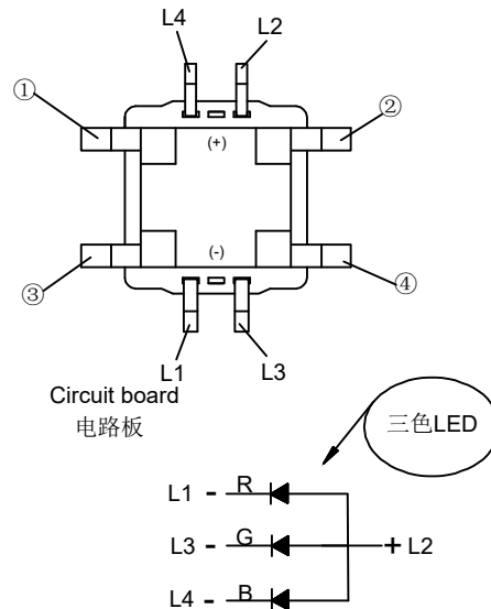
PCB. Installation diagram PCB. 安装示意图
