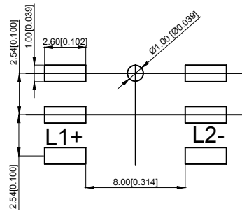
Installation diagram 安装示意图
