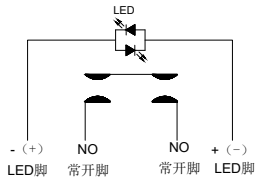
Schematic Diagram 电气原理图
