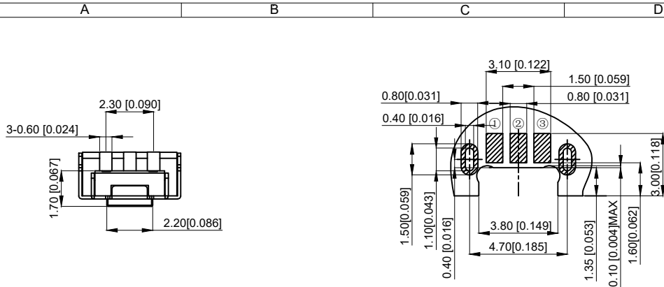
PCB.安装图
