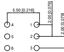
印制线路板
