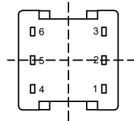
向视图
