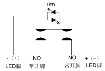
Schematic Diagram 电气原理图
